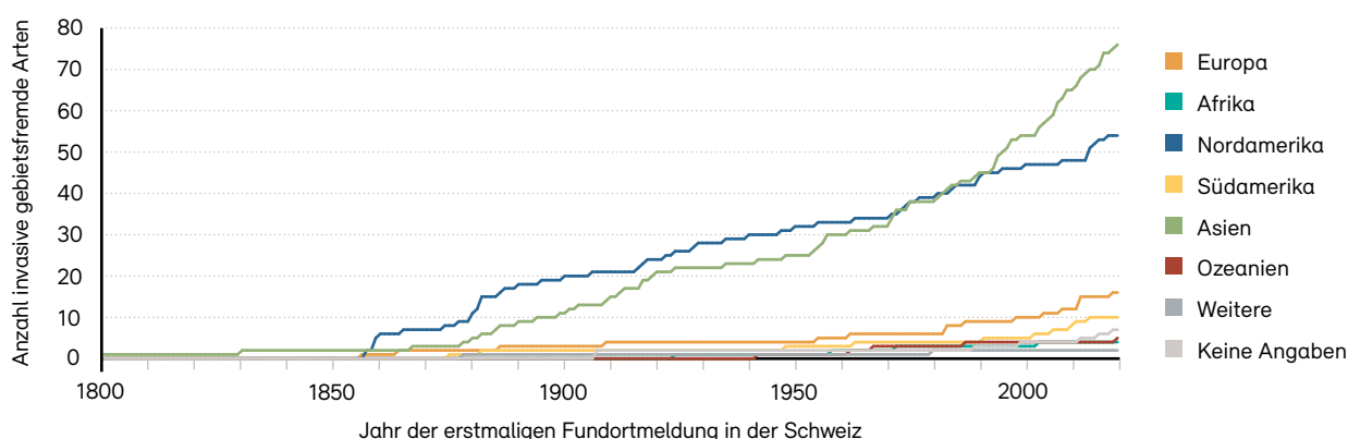
Abb. 9: Zeitliche Entwicklung und Herkunftsregionen der invasiven gebietsfremden Arten
